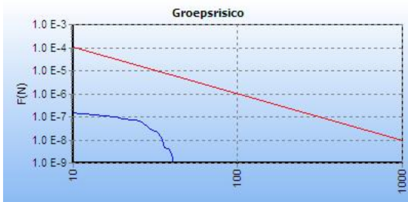
Figuur 5.1 FN curve voor N-560-03 van N.V. Nederlandse Gasunie voor de kilometer tussen stationing 11330.00 en stationing 12330.00
