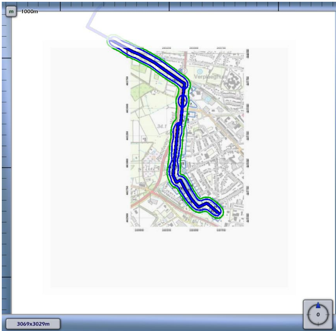
Figuur 3.1 Plaatsgebonden risico voor N-560-03 van N.V. Nederlandse Gasunie
