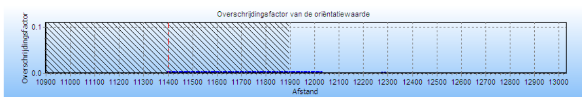
Figuur 4.1 Groepsrisico screening voor N-560-03 van N.V. Nederlandse Gasunie
