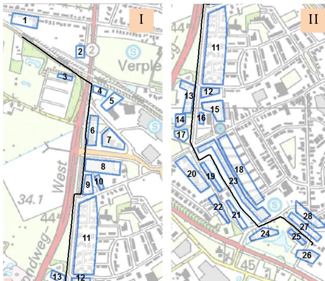
Figuur 5. Bevolkingsgebieden Carola. Links (I) betreft de noordelijke helft, rechts (II) betreft de zuidelijke helft. De zwarte lijn betreft het beschouwde deel van de aardgasleiding.
