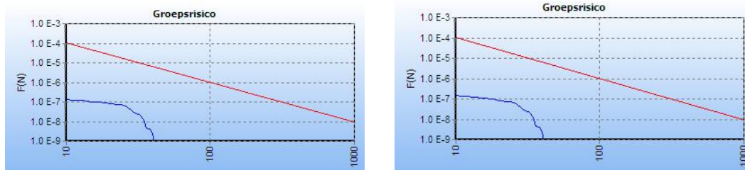
Figuur 3. Groepsrisicocurve huidige bestemming (links) en nieuwe bestemming (rechts)
