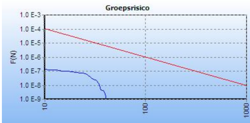
Figuur 5.1 FN curve voor N-560-03 van N.V. Nederlandse Gasunie voor de kilometer tussen stationing 10900.00 en stationing 11900.00
