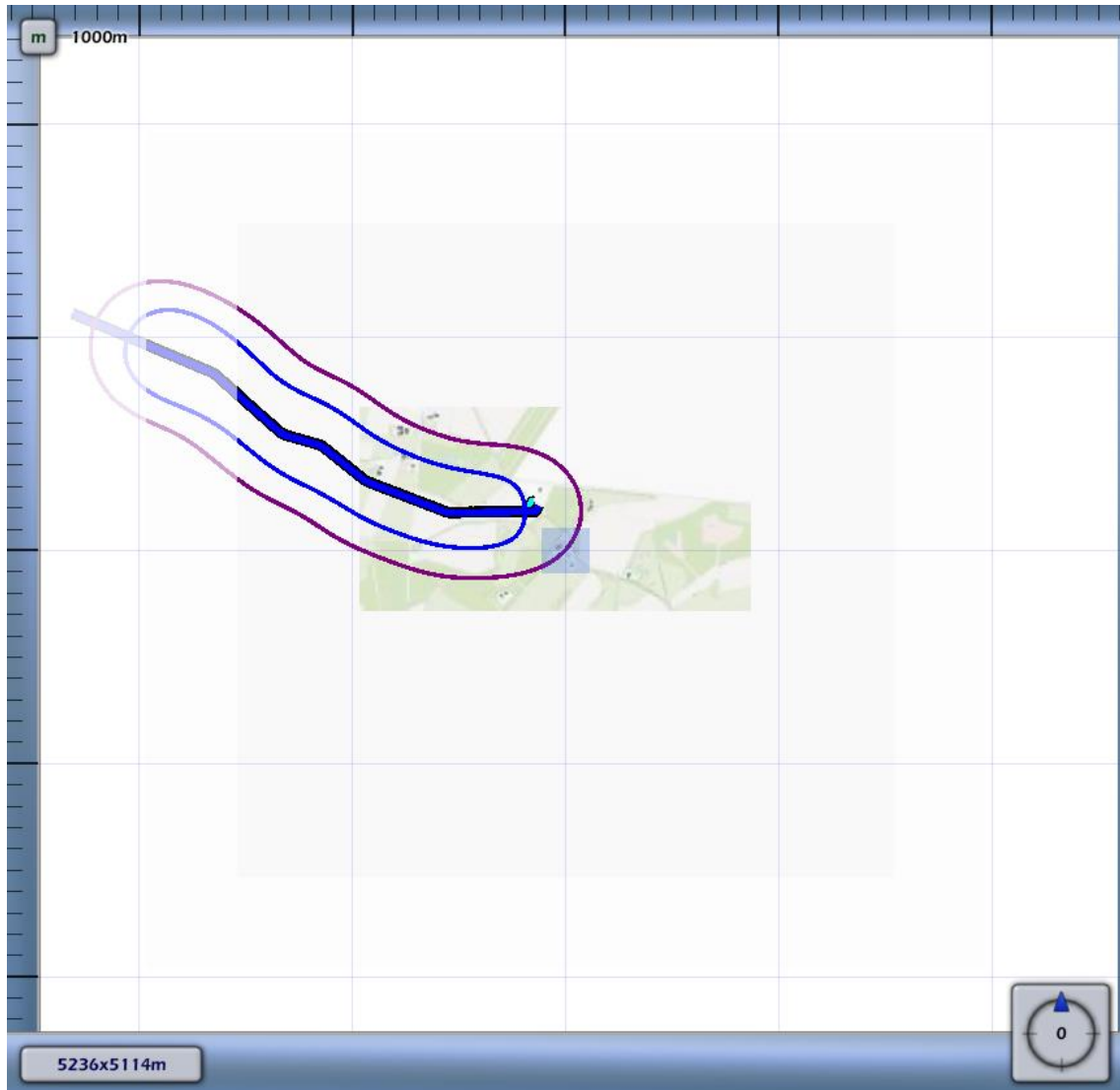
3.2 Figuur 3.2 Plaatsgebonden risico voor leiding-A-628-deel-1 van N.V. Nederlandse Gasunie
