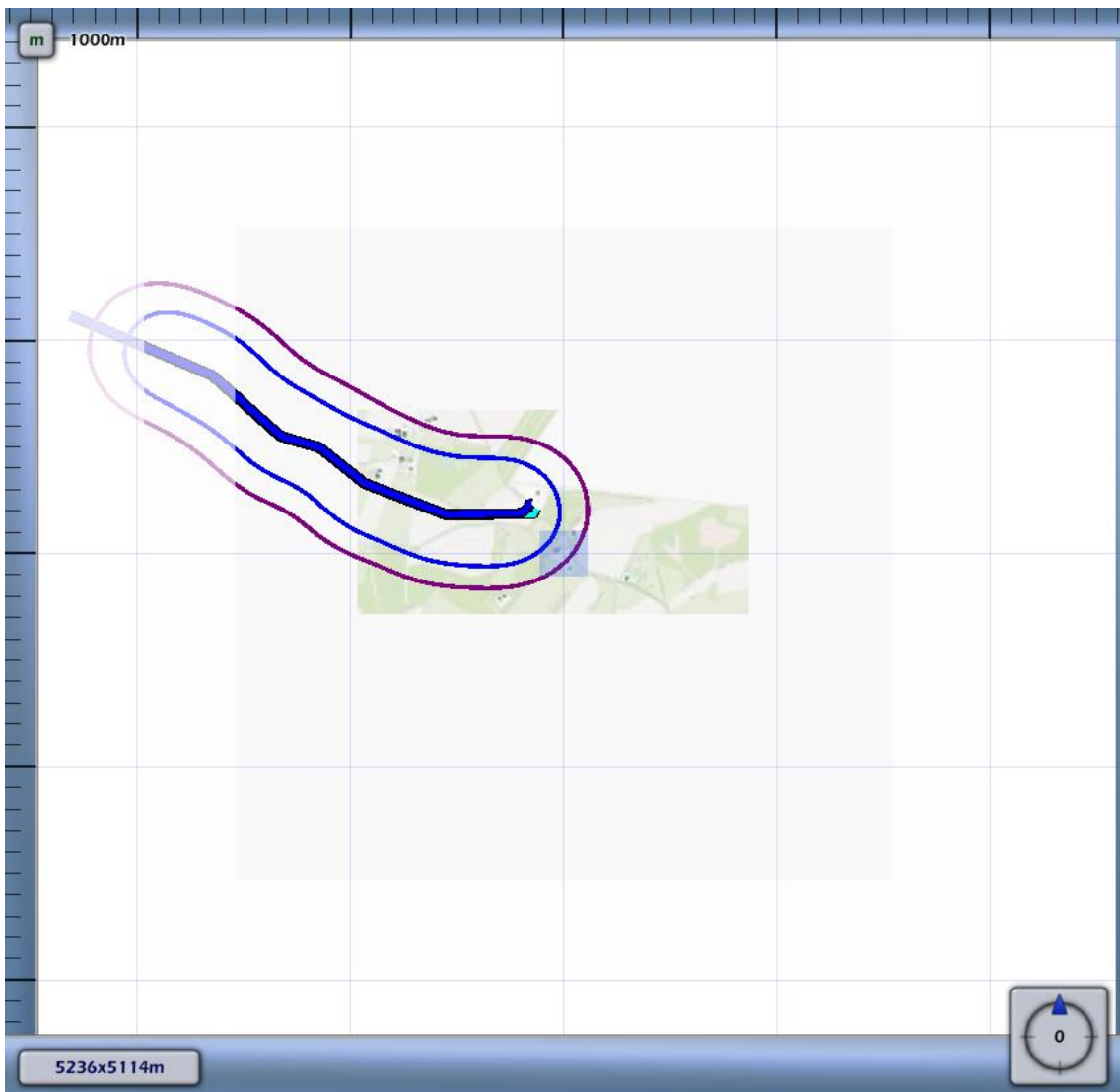
3.1 Figuur 3.1 Plaatsgebonden risico voor leiding-A-579-deel-1 van N.V. Nederlandse Gasunie
