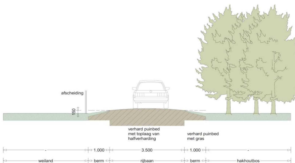
Profieldoorsnede toegangsweg
