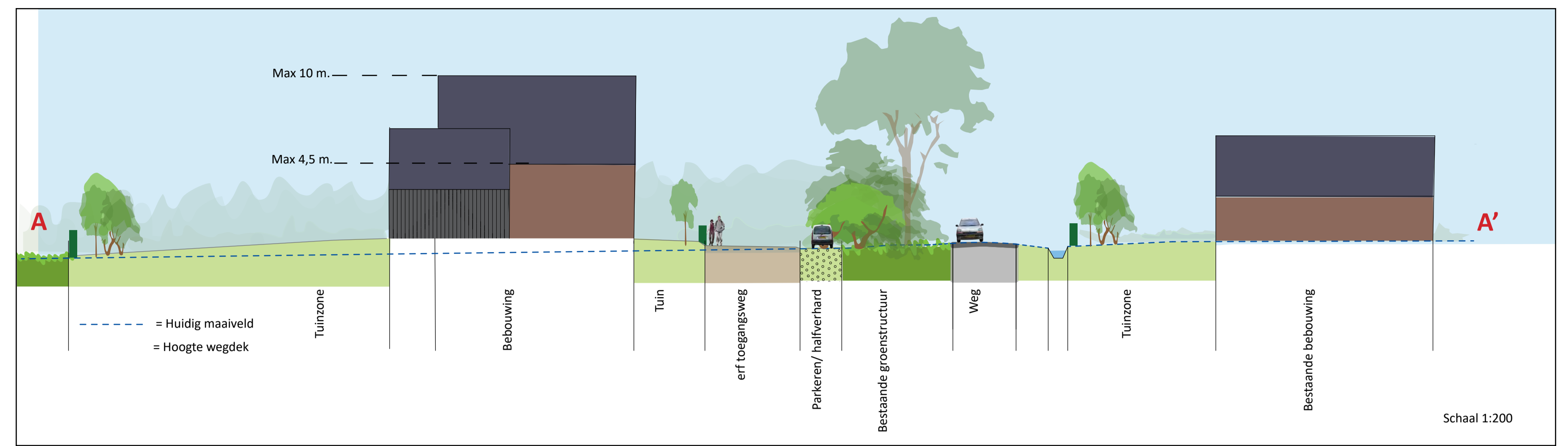
Dwarsprofiel A-A'
