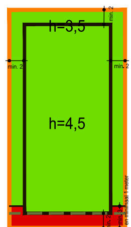
Hoofdgebouw
